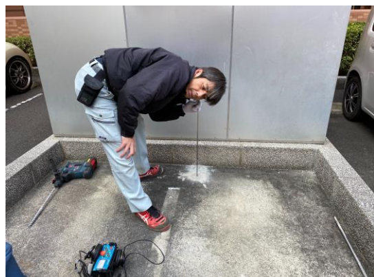
地中音聴で漏水による噴射音を確認 漏水箇所に確定し調査終了
