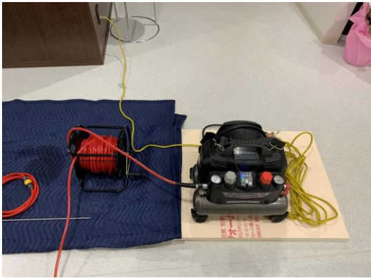
コンプレッサーを排水口に接続し、圧縮空気を充填
