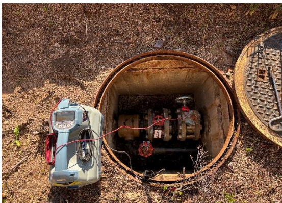
鉄管探知器による管路調査
