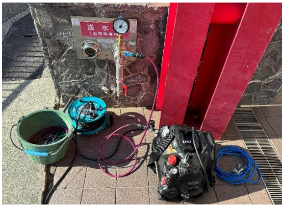
コンプレッサーを送水口に接続しエアを充填
